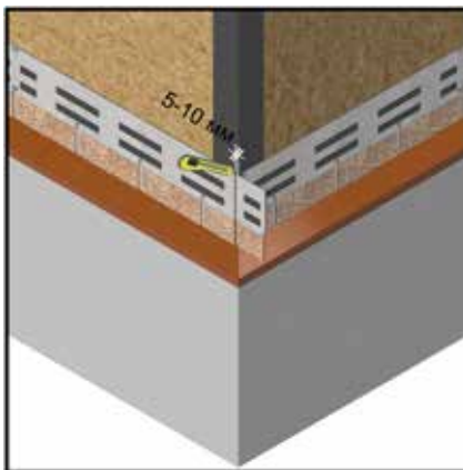
Рис. 14 Подрезка фасадной плитки при подходе к углам.
